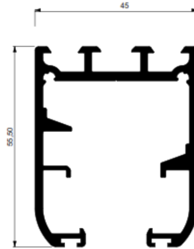
PERFIL MARCO SUPERIOR
