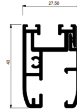
PERFIL HOJA-EMBELECEDOR
