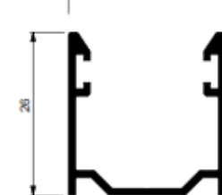
PERFIL LATERAL "U"
