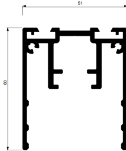
PERFIL COMPENSADOR
