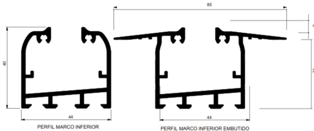
PERFIL MARCO INFERIOR EMBUTIDO
